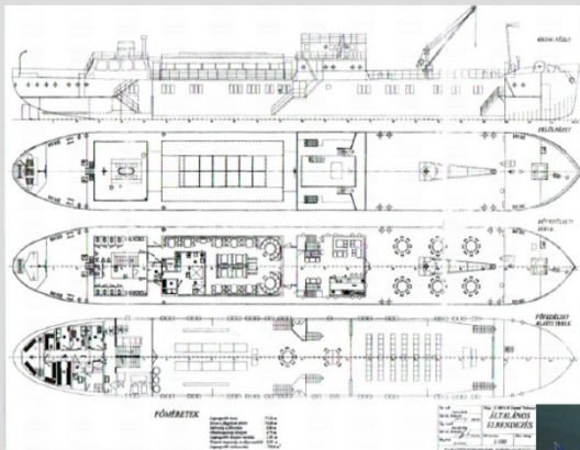
átalakítás tervei (2011)
